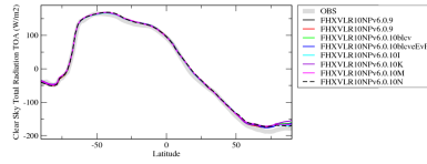
rttcson
