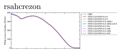
rsahzon
