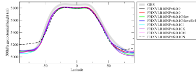
zg500zn
