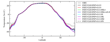
taszn
