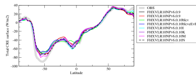
crettszon
