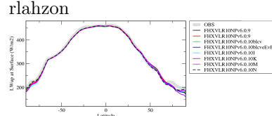
lsruon
