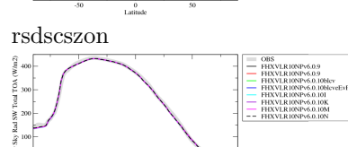
rsdszon
