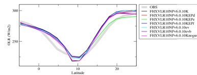
rlutzn
