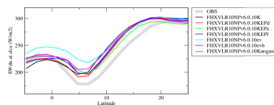
rdsdzon
