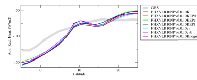
rahzn
