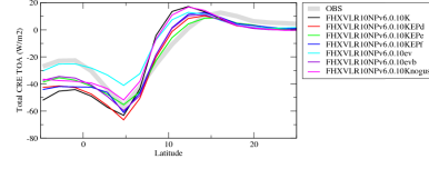
crettzon
