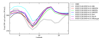
rdszn
