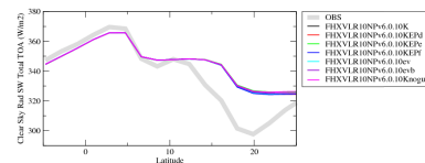
rsttcszon
