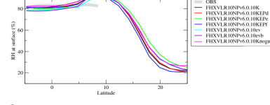
hurszon
