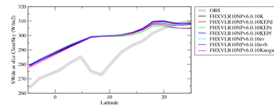
rdsdcszon
