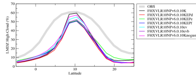
chlzon
