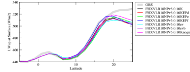
rlszon
