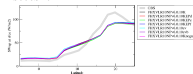
rsuszn
