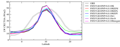
creltzon
