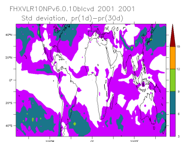
FHXVLR10NPv6.0.10blev_2001_2001_hf
