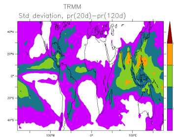
TRMM_is
