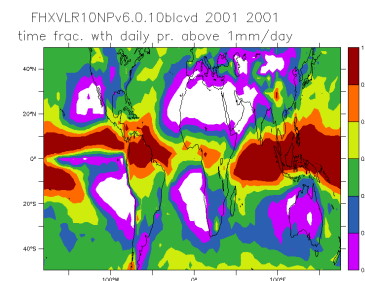
FHXVLR10NPv6.0.10blev_2001_2001_nd
