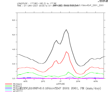
FHXVLR10NPv6.0.10blcvfEvP
