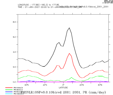
FHXVLR10NPv6.0.10blevd_2001_2001_zon
