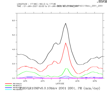
FHXVLR10NPv6.0.10blev_2001_2001_zon
