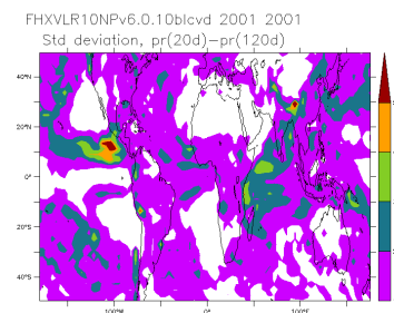
FHXVLR10NPv6.0.10blev_2001_2001_is
