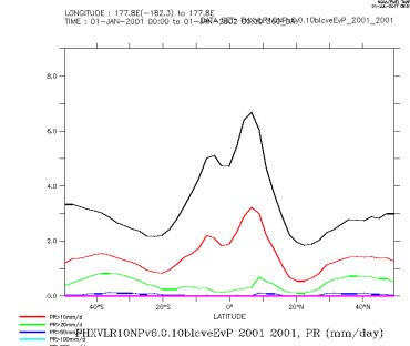
FHXVLR10NPv6.0.10blcveEvP
