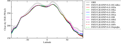
rlutscszon
