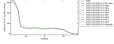
rsutsczon
