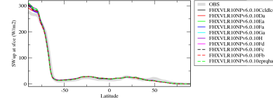
rsuscsczon
