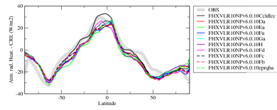
rahcrezon
