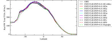
rsttsczon
