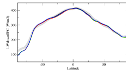
rldscszon
