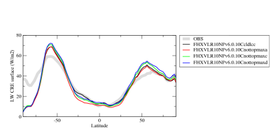
cllzon
