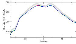
rlutscszon
