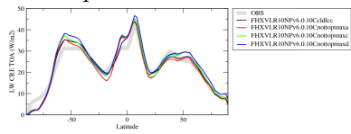
crelcalipsozon
