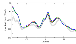
rahzon
