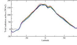
rsutscszon
