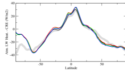
rlahcrezon
