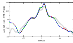
rahcrezon
