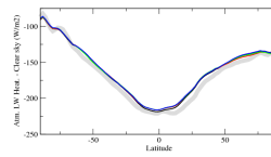
rlahcszon
