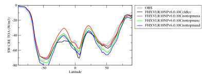
crelcalipsozon
