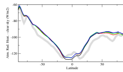
rahcszon
