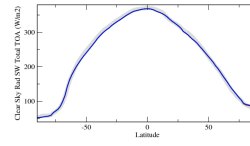
rsdscszon
