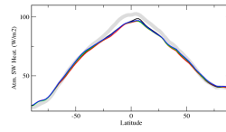
rsahcszon
