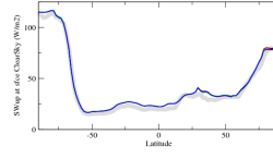
rsttsczon
