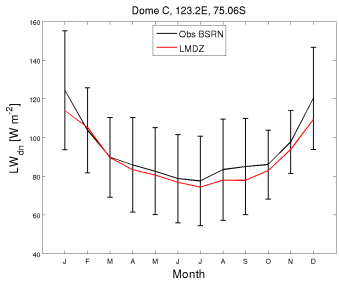
LWdnSFC_DC_FHXVLR10NPv6.0.10C_2001_2008
