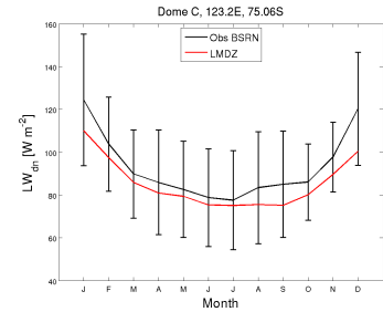
LWdnSFC_DC_FHXVLR10NPv6.0.10epqrh_2001_2008
