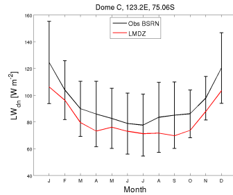
LWdnSFC_DC_FHXVLR10NPv6.0.10_2001_2008
