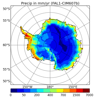
precipSH-FAL1-CIM607b
