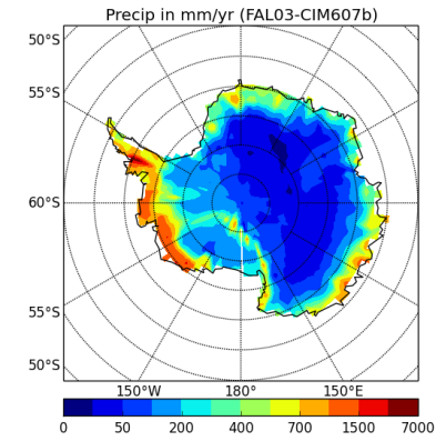
precipSH-FAL03-CIM607b
