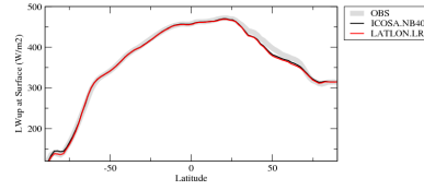
rldzon
