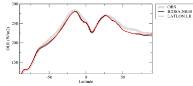
rlutszon
