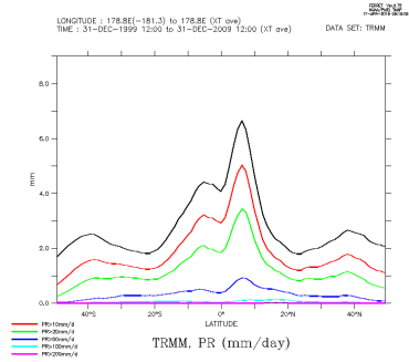
TRMM_zon
