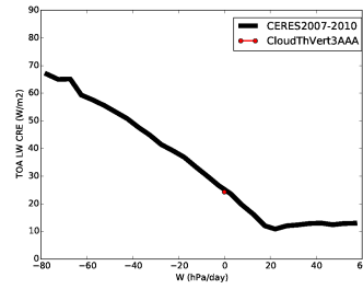
cretl_CldThT0
