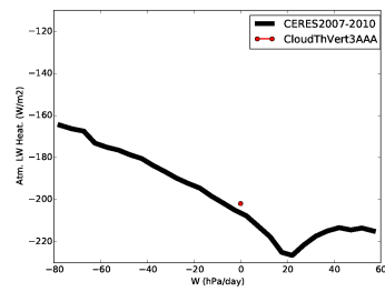
ralah_CldThT0
