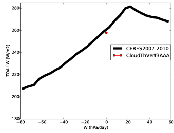
rlut_CldThT0
