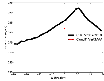
rlutcs_CldThT0
