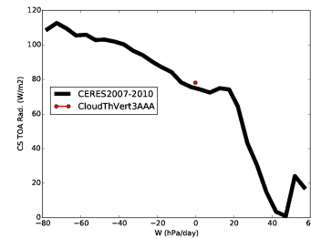
rttcs_CldThT0
