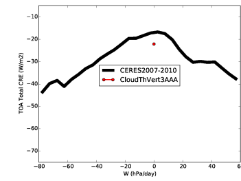
crettt_CldThT0
