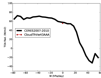
rtt_CldThT0
