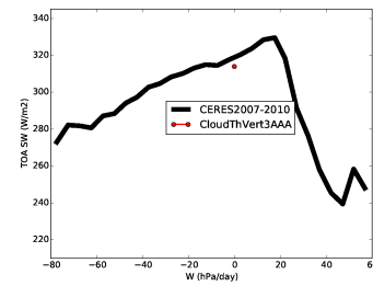
rstt_CldThT0
