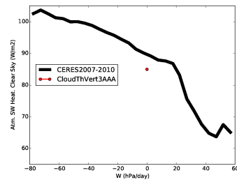
rsahcs_CldThT0
