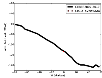
rah_CldThT0
