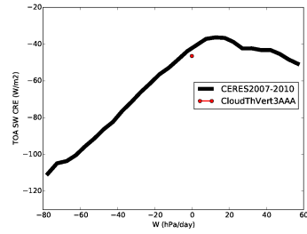
crest_CldThT0
