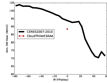
rsah_CldThT0
