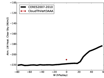
ralahcs_CldThT0
