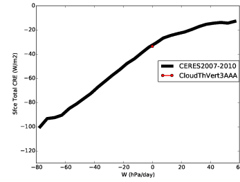
cretst_CldThT0
