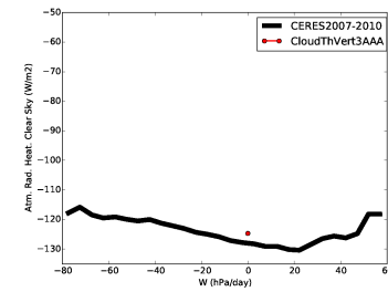
rahcs_CldThT0
