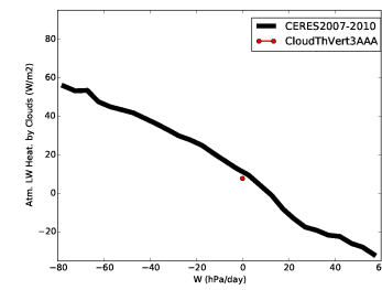
ralahcre_CldThT0
