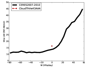
crels_CldThT0
