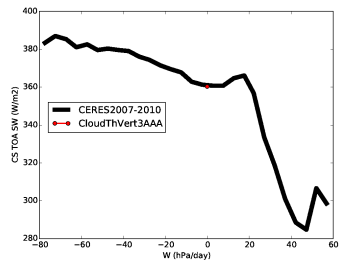
rsttcs_CldThT0
