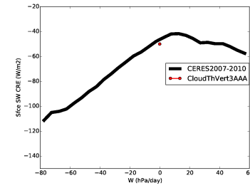
cress_CldThT0
