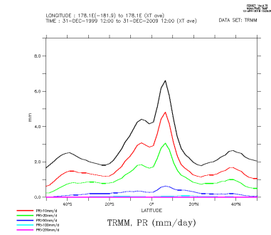
TRMM_zon
