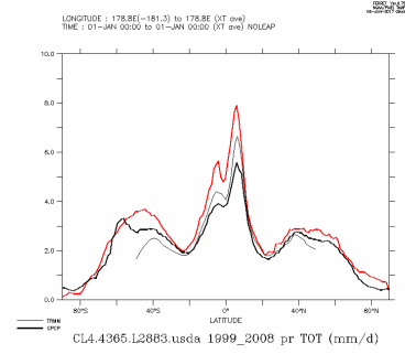
CL4.4365.L2883.usda.1999_2008_tot
