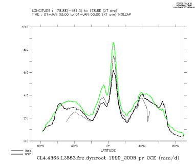
CL4.4365.L2883.frz.dynroot.1999_2008_oce
