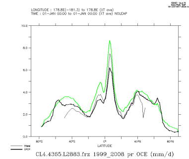
CL4.4365.L2883.frz.1999_2008_oce
