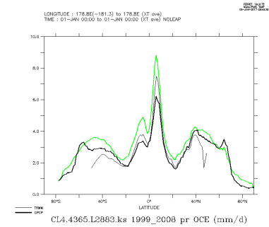
CL4.4365.L2883.ks.1999_2008_oce
