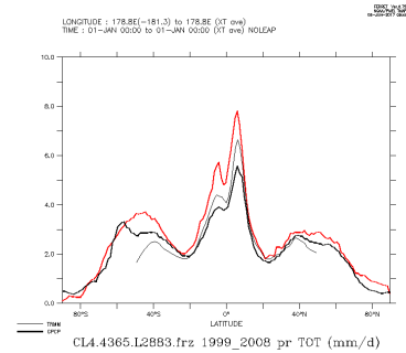
CL4.4365.L2883.frz.1999_2008_tot
