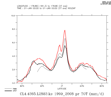
CL4.4365.L2883.ks.1999_2008_tot
