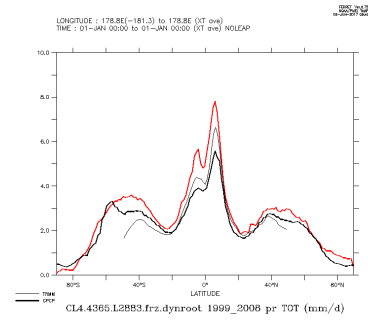
CL4.4365.L2883.frz.dynroot.1999_2008_tot
