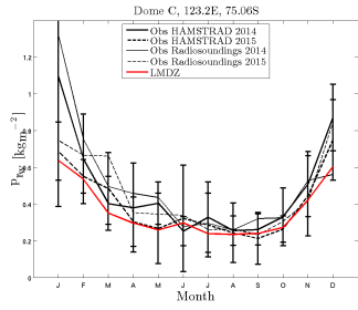
prw_DC LMDZOR3607b_1980_1989
