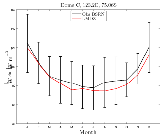
LWdn_DC LMDZOR01alb_1980_1989
