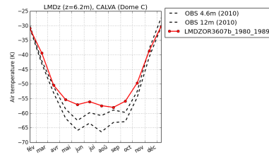
tempDC-LMDZOR3607b_1980_1989
