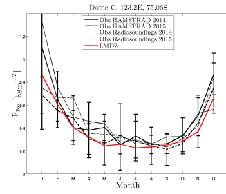
prw_DC LMDZOR01alb_1980_1989
