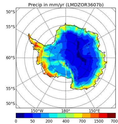
precipSH-LMDZOR3607b
