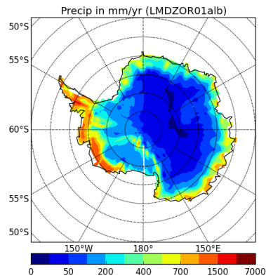
precipSH-LMDZOR1alb
