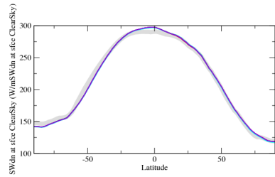
albszon
