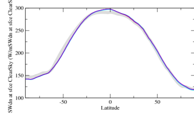
clmcalipsozon
