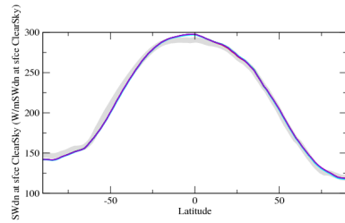
rsahzon
