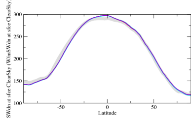
rsuteszon
