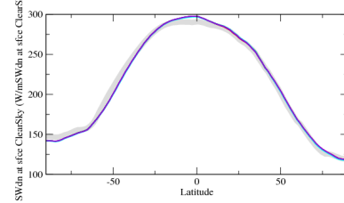
crelszon
