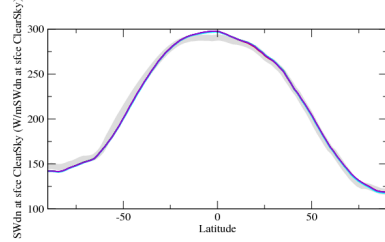
rstszon
