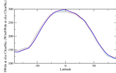
rttzn
