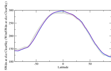
przon
