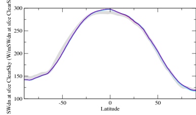
clcalipsozon
