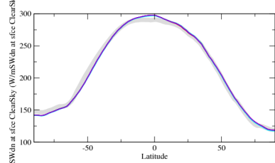
hfszonzon
