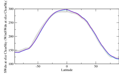
rsdszon
