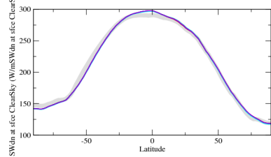
rlutcszon
