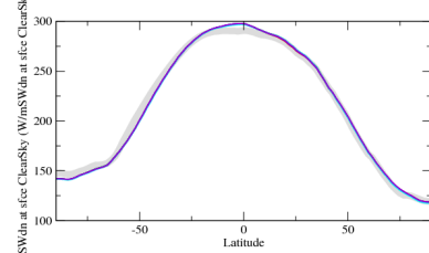
hffszonzon
