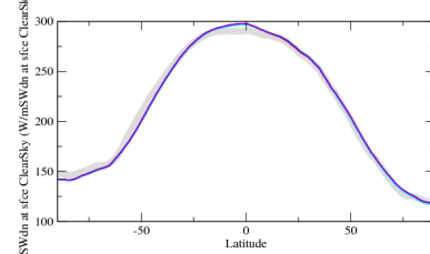
hurszonzon
