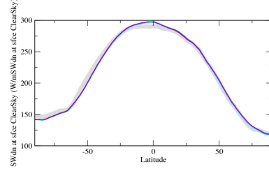
rsttcszon
