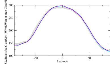
crettzn
