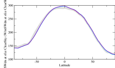
cretszon
