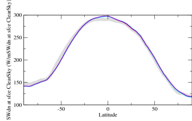
rttcszon
