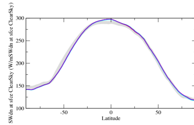
pslzon
