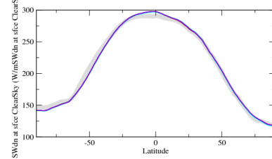
rsahcrezon
