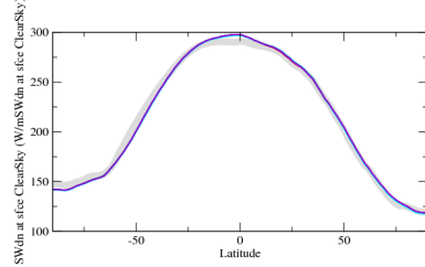
rstzn
