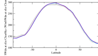
rahzon
