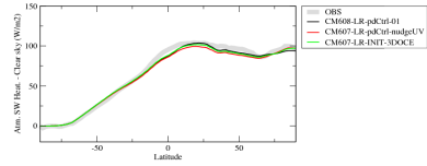
rsahcszone
