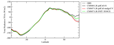
rttzone
