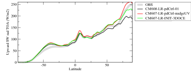
rsutzone
