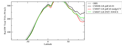
rsttzone
