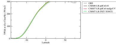
rsdscszone
