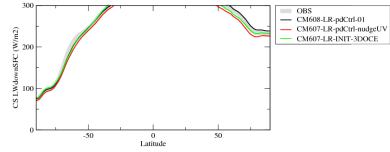
rldscszone
