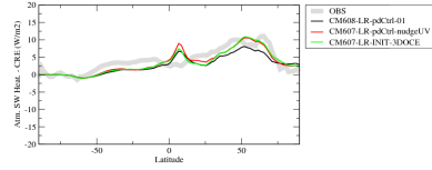
rsahcrezone
