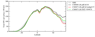
rstsczone
