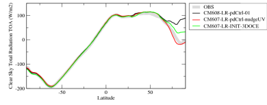
rttcszone
