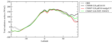
rtsczone
