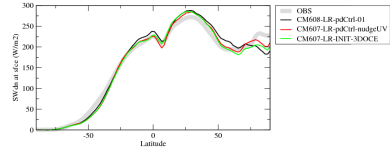
rsdsczone
