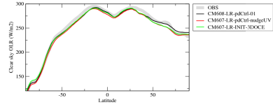
rlutcszone
