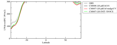
rldsczone
