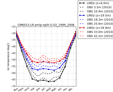
tempDC_CM6015-LR-amip-split-G-02_1999_2008
