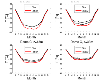
temp_DC_CM6015-LR-amip-split-G-02_1999_2008
