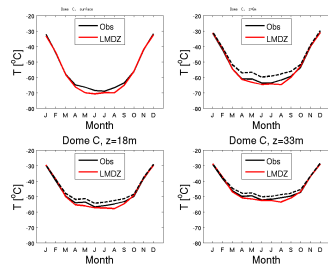
temp_DC_CM6015-LR-amip-split-02_1999_2008
