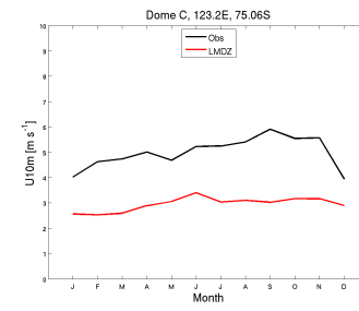
prw_DC_CM6015-LR-amip-ttop-G-02_1999_2008
