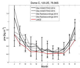
prw_DC_CM6015-LR-amip-split-G-02_1999_2008
