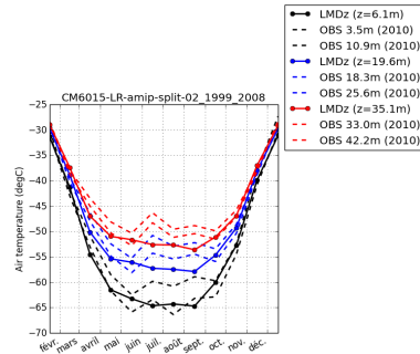
tempDC_CM6015-LR-amip-split-02_1999_2008
