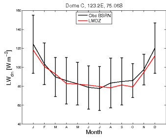
LWdnSFC_DC_LMDZOR6.0.12split.NUD_2000_2009
