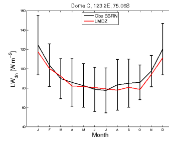
LWdnSFC_DC_LMDZOR6.0.12split.NEWG.NUD_2000_2009
