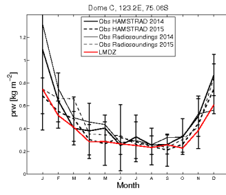
prw_DC_LMDZOR6.0.12split.NUD_2000_2009
