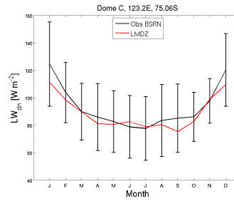
LWdnSFC_DC_LMDZOR6.0.12.NOGUST_1995_2004
