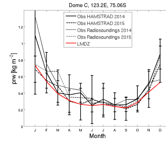
prw_DC_LMDZOR6.0.12_1995_2004
