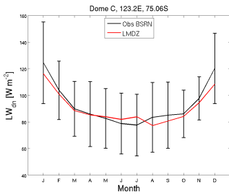
LWdnSFC_DC_LMDZOR6.0.12.NOZ0_1995_2004
