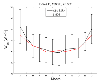
LWdnSFC_DC_LMDZOR6.0.12.NOZ0.MWS_1995_2004
