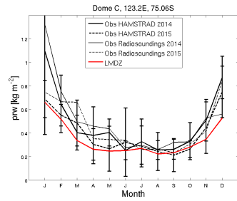
prw_DC_LMDZOR6.0.12.NG_1995_2004
