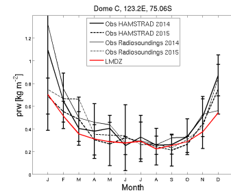
prw_DC_LMDZOR6.0.12.NOZ0_1995_2004
