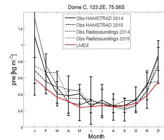
prw_DC_LMDZOR6.0.12.NOZ0.MWS_1995_2004
