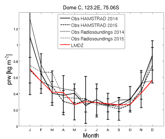
prw_DC_CPL6.0.12.1950_1959
