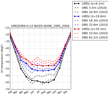
tempDC-LMDZOR6-0-12-NOZ0-QH98_1995_2004
