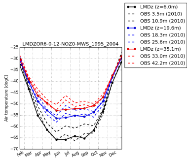
tempDC-LMDZOR6-0-12-NOZ0-MWS_1995_2004
