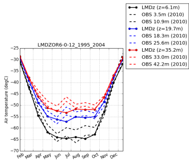
tempDC-LMDZOR6-0-12_1995_2004
