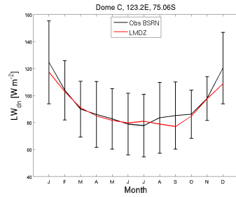
LWdnSFC_DC_LMDZOR6.0.12_1995_2004
