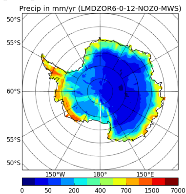
precipSH-LMDZOR6-0-12-NOZ0-MWS
