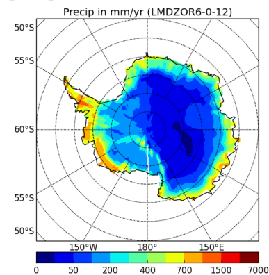
precipSH-LMDZOR6-0-12
