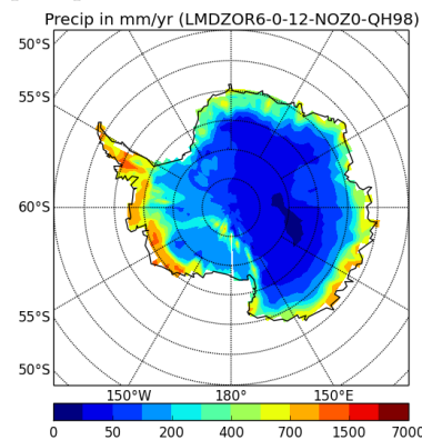
precipSH-LMDZOR6-0-12-NOZ0-QH98
