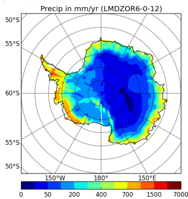
precipSH-LMDZOR6-0-12
