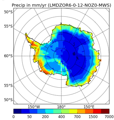
precipSH-LMDZOR6-0-12-NOZ0-MWS
