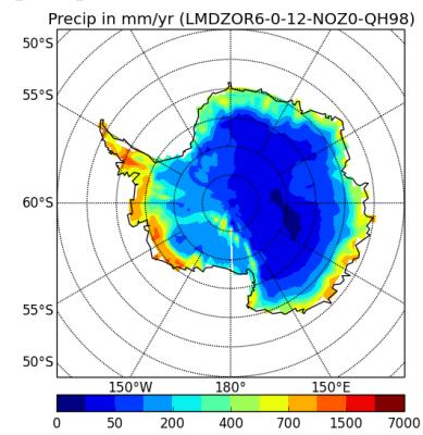
precipSH-LMDZOR6-0-12-NOZ0-QH98
