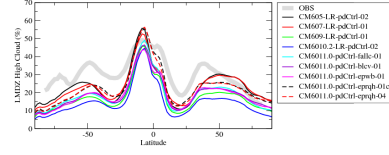
rsttsczone
