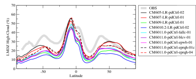
rlahcrezon
