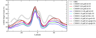
rttsczon
