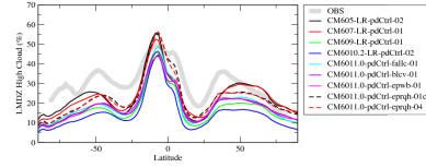
rlusczone
