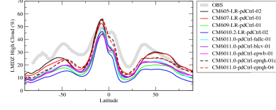
sttszone
