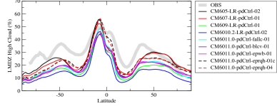
alhcalipsozon
