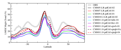
tauvzon
