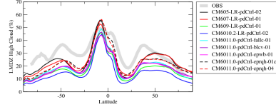
alhcalipsozon
