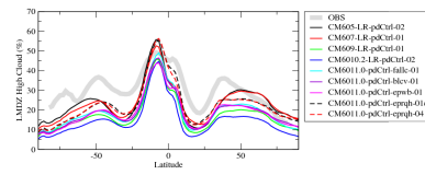
alhcalipsozon
