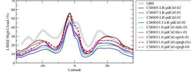
rsttsczon
