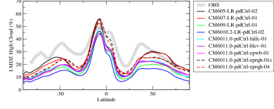
rttcszon
