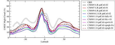
rsahcszon
