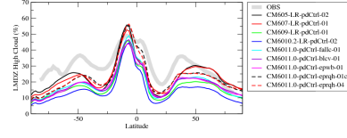
rttsczone
