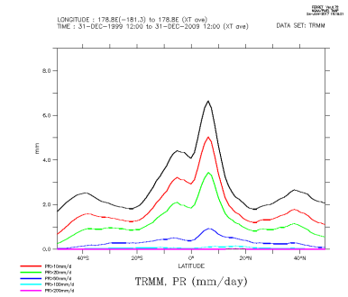
TRMM_zon
