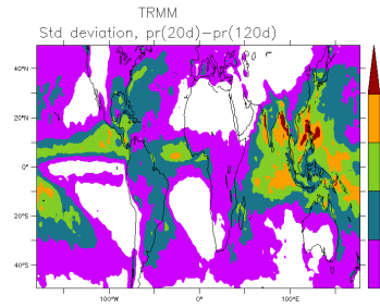
TRMM_ls
