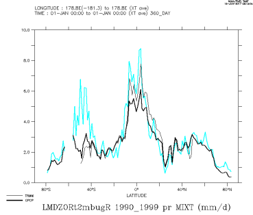
LMDZORt2mbugR_1990_1999_mix
