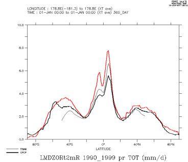
LMDZORt2mR_1990_1999_tot
