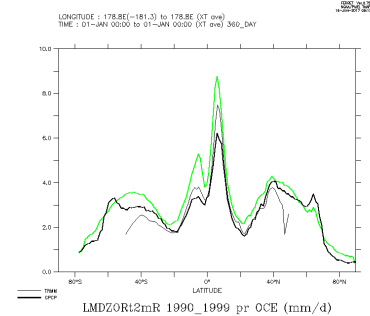
LMDZORt2mR_1990_1999_oce
