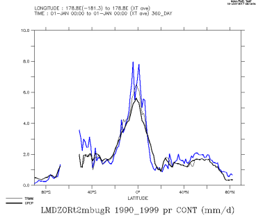
LMDZORt2mbugR_1990_1999_con
