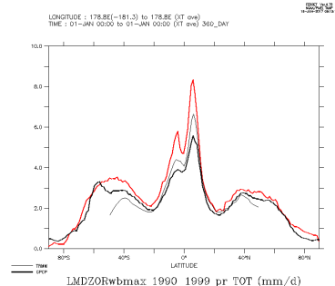
LMDZORwbmax_1990_1999_tot
