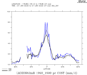
LMDZORt2mR_1990_1999_con
