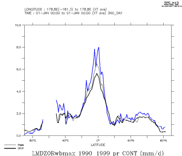
LMDZORwbmax_1990_1999_con
