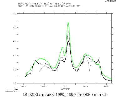
LMDZORt2mbugR_1990_1999_oce
