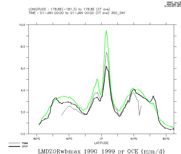
LMDZORwbmax_1990_1999_oce
