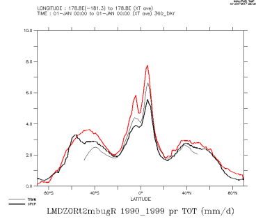
LMDZORt2mbugR_1990_1999_tot
