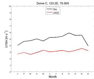
wind10m_DC_BORNEFHv2_1980.1984
