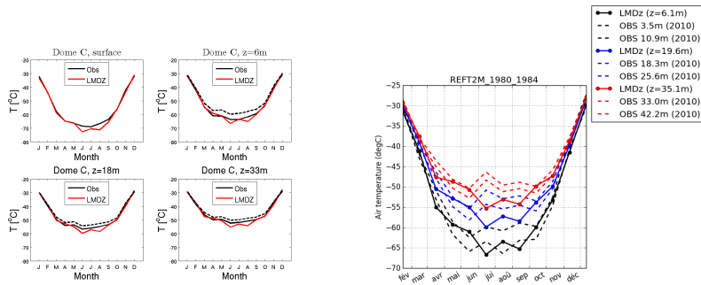
temp_DC_REFT2M_1980.1984
