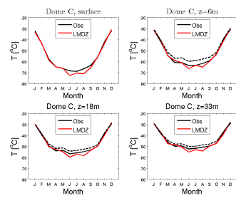
temp_DC_BORNEFHv2_1980.1984
