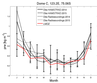
prw_DC_BORNEFHv2_1980.1984
