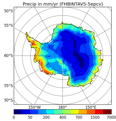
precipSH-FHBINTAV5-5epcv
