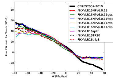
rlahcre_BEST5
