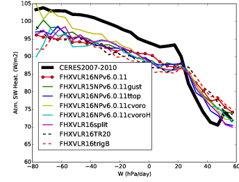
rsah_BEST5
