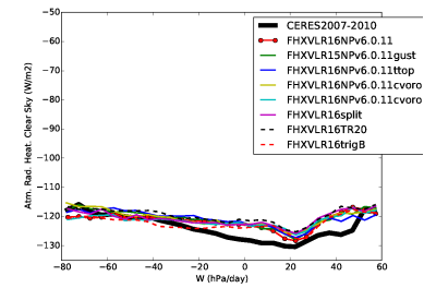
rahcs_BEST5
