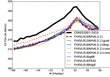
rlutcs_BEST5
