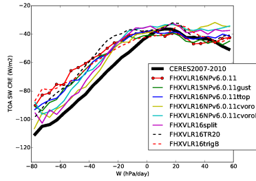
crest_BEST5
