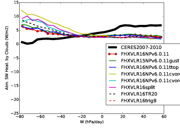
rsahre_BEST5
