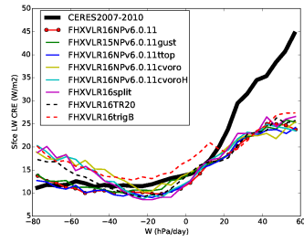
crels_BEST5
