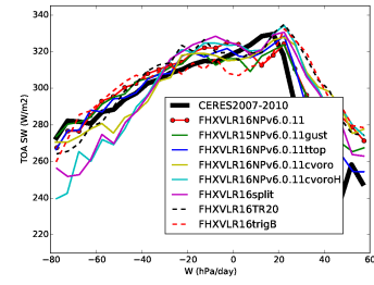
rstt_BEST5
