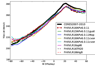
rlut_BEST5
