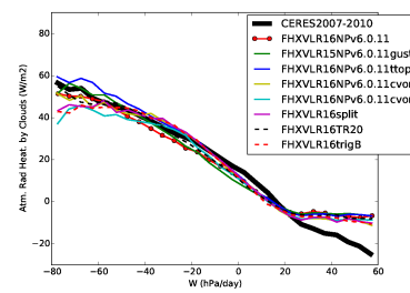
rahcre_BEST5
