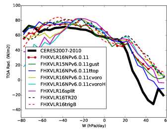
rtt_BEST5
