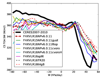
rsttcs_BEST5
