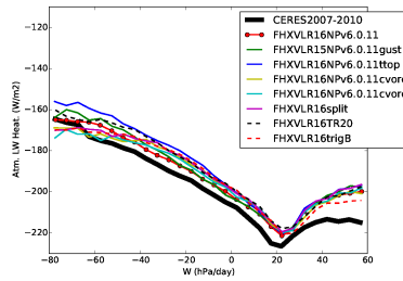
rlah_BEST5
