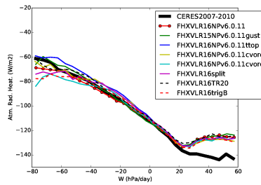
rah_BEST5
