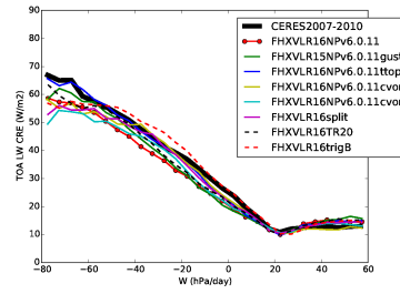
crelt_BEST5
