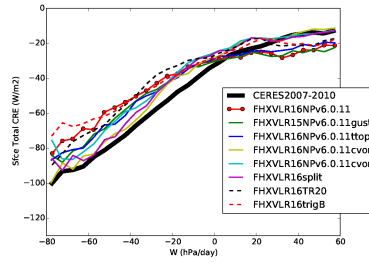
crets_BEST5
