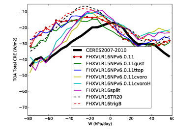
crett_BEST5
