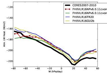
ralah_BEST1
