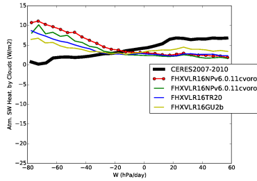
rsahre_BEST1
