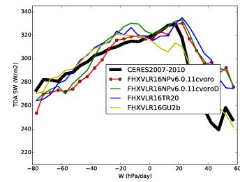
rstt_BEST1
