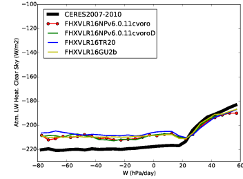
ralahcs_BEST1
