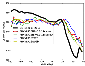
rsttcs_BEST1
