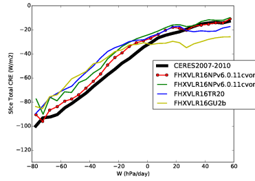
cretst_BEST1
