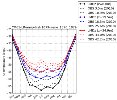
tempDC_CM61-LR-amip-hist-1879-irene.1870-1879
