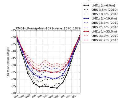
tempDC_CM61-LR-amip-hist-1871-irene_1870_1879
