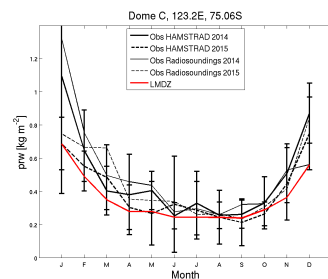
prw_DC_CM61-LR-amip-hist-1872-irene_1870_1879
