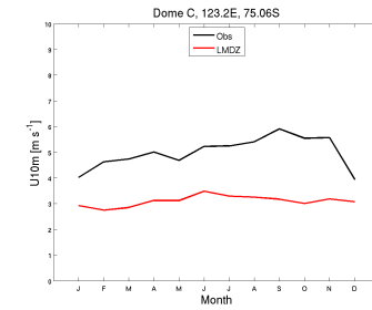
prw_DC_CM61-LR-amip-hist-1878-irene.1870-1879
