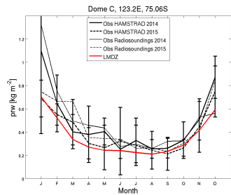
prw_DC_CM61-LR-amip-hist-1871-irene_1870_1879
