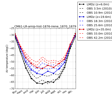
tempDC_CM61-LR-amip-hist-1876-irene_1870_1879
