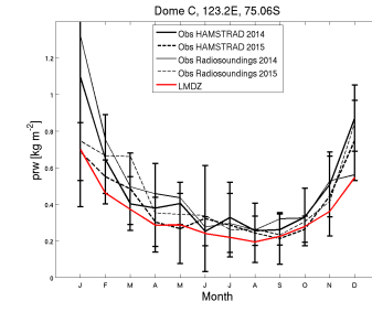
LWdnSFC_DC_CM61-LR-amip-hist-1874-irene_1870_1879
