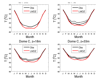
temp_DC_CM61-LR-amip-hist-1871-irene_1870_1879
