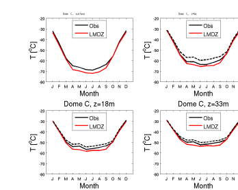
temp_DC_CM61-LR-amip-hist-1872-irene_1870_1879
