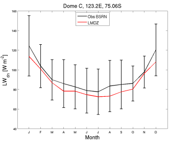
LWdnSFC_DC_CM61-LR-amip-hist-1877-irene.1870-1879
