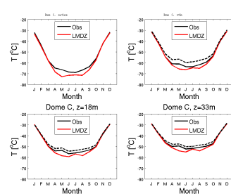
temp_DC_CM61-LR-amip-hist-1876-irene_1870_1879
