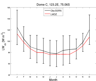
LWdnSFC_DC_CM61-LR-amip-hist-1872-irene_1870_1879
