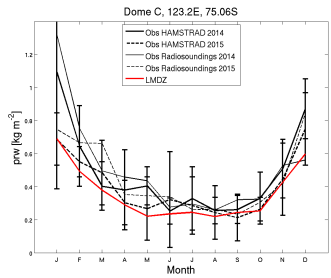
prw_DC_CM61-LR-amip-hist-1876-irene.1870-1879
