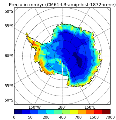
precipSH-CM61-LR-amip-hist-1872-irene
