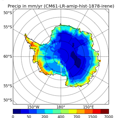
precipSH-CM61-LR-amip-hist-1878-irene
