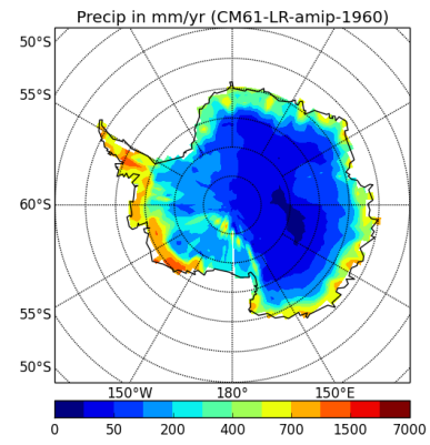
precipSH-CM61-LR-amip-1960
