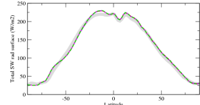
rstsczon
