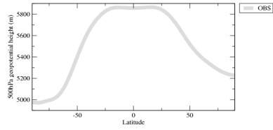
zg500zon
