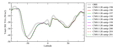
cretzon
