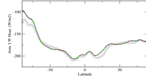
rlahczon
