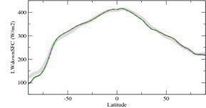
rldsczon
