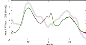
rsahcrezon
