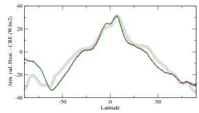
rahcrezon
