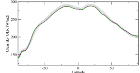
rlutcszon
