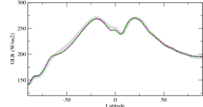
rlutczon
