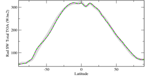
rsttzo
