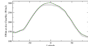
rsdscszo
