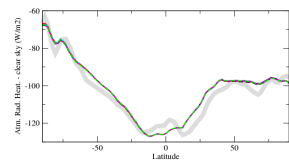
rahczon
