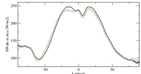
rsdsczon
