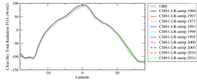
rttsczon
