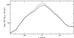
rsahczon
