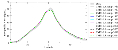
prwzon
