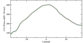
rldscszo
