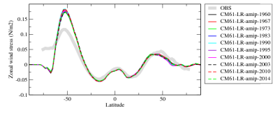
tauzon
