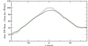
rsahcszon
