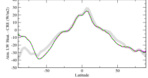
ralahcrezon
