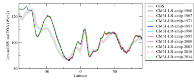
rsutzon
