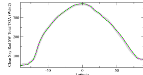
rsttcszo
