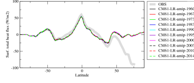
hfmszon
