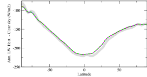
rlahcszon
