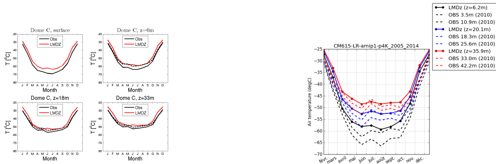
temp_DC_CM615-LR-amip1-p4K_2005_2014
