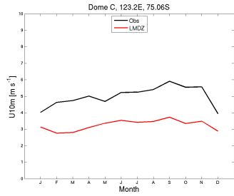
wind10m_DC_CM615-LR-amip1-p4K_2005_2014
