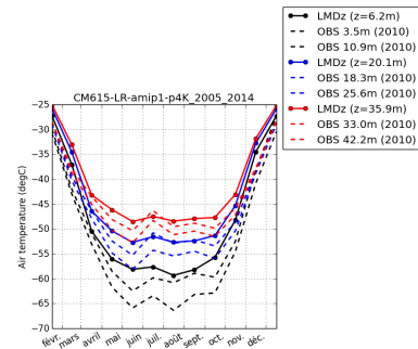
tempDC_CM615-LR-amip1-p4K_2005_2014
