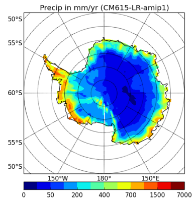
precipSH-CM615-LR-amip1
