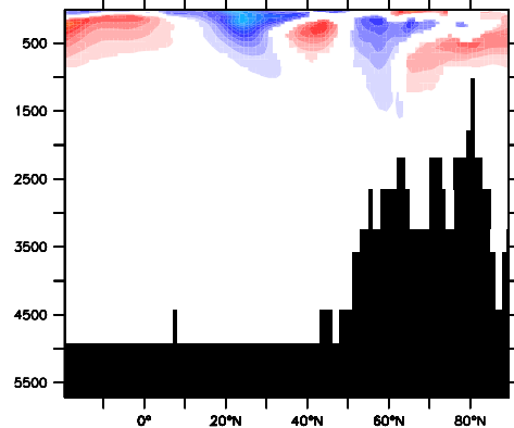
d) EcEarth
