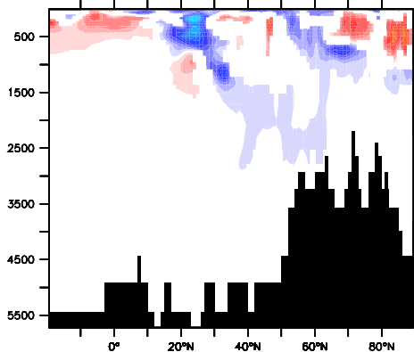
c) MPI-ESM
