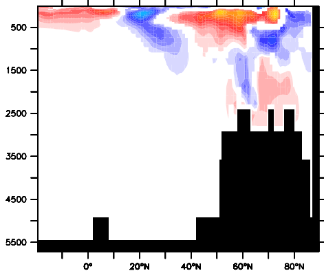
c) MPI-ESM
