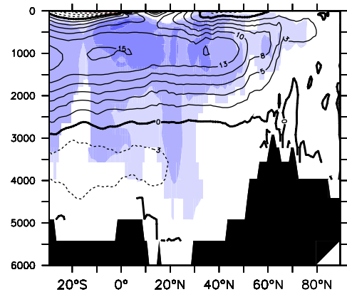
c) MPI-ESM
