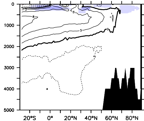
b) IPSLCM5
