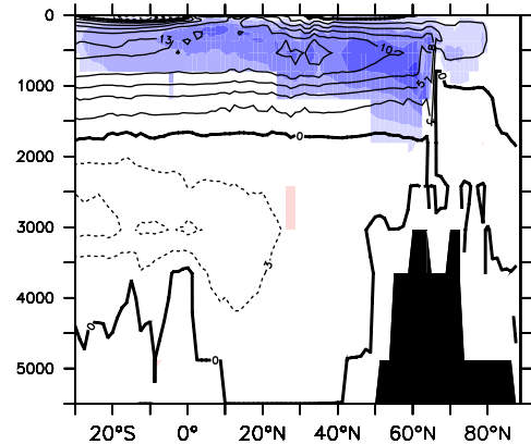
c) MPI-ESM
