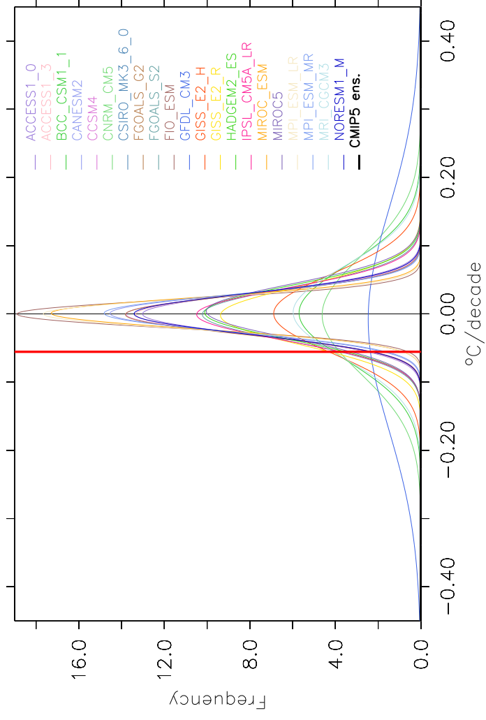
b) SST 36-yr trend: piControl
