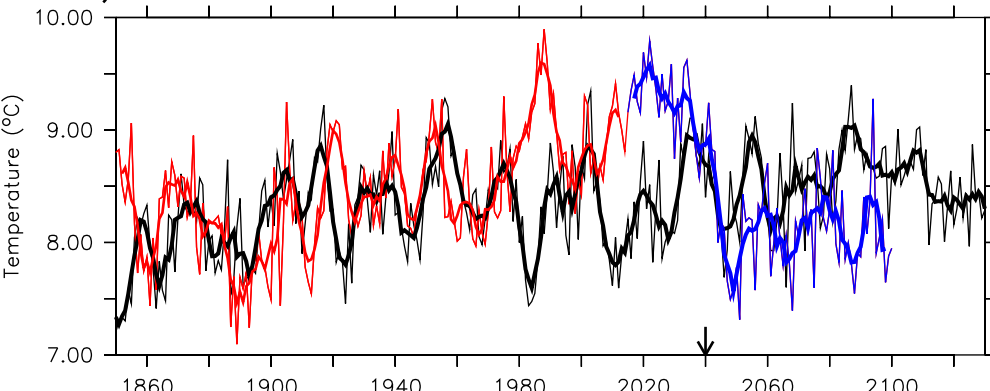
c) NorESM2-LM
