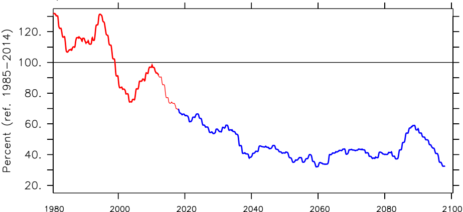
c) NorESM2-LM
