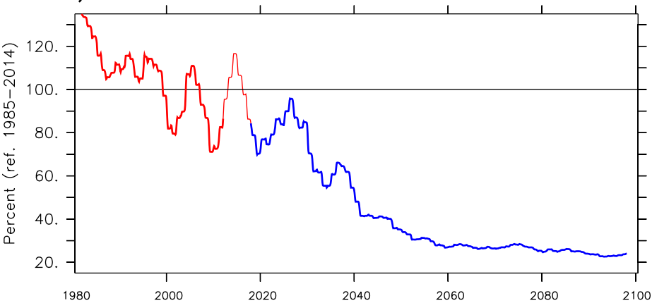
c) NorESM2-LM
