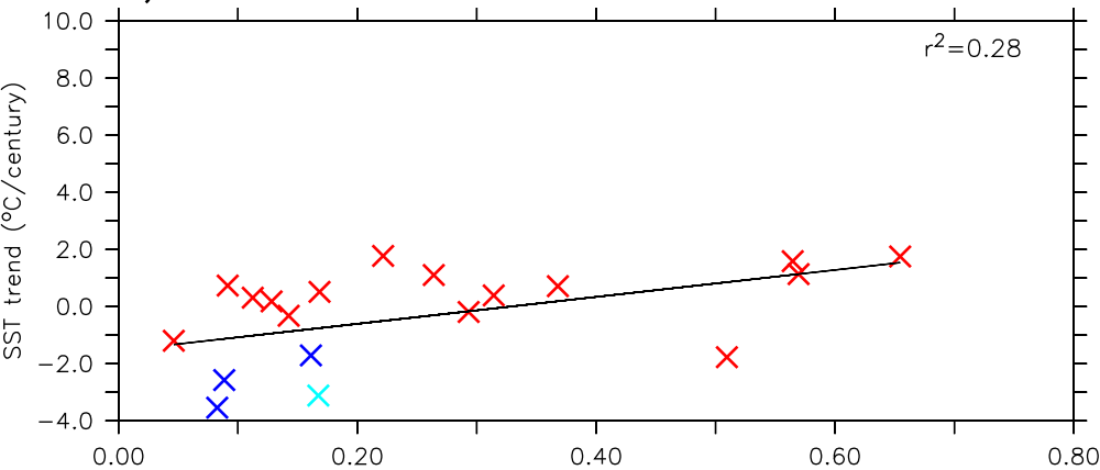
b) SSP245
