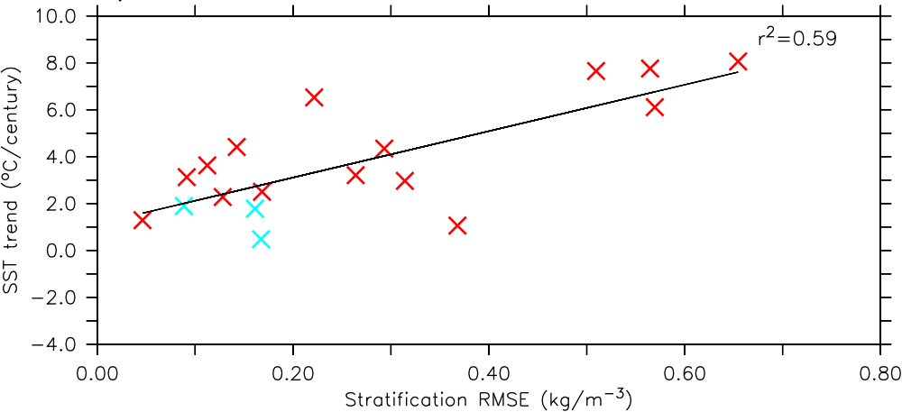
c) SSP585
