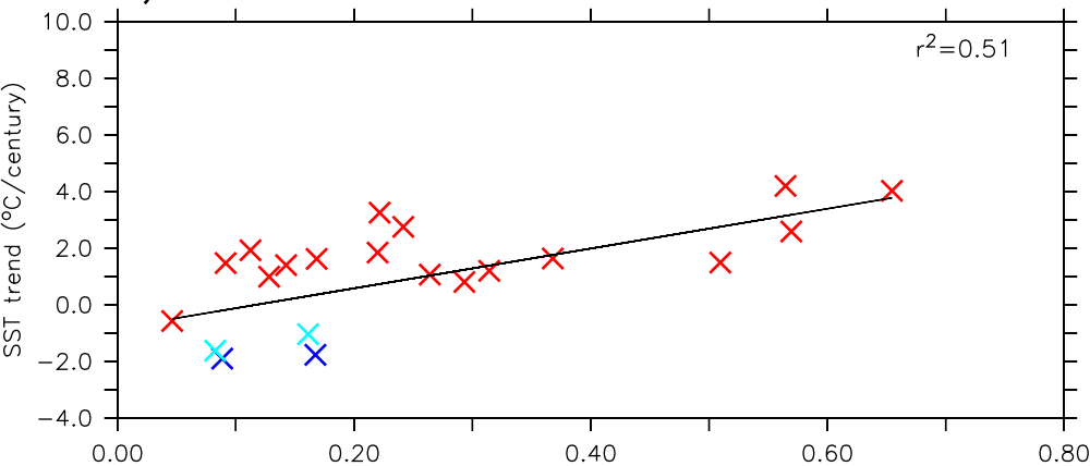
c) SSP585
