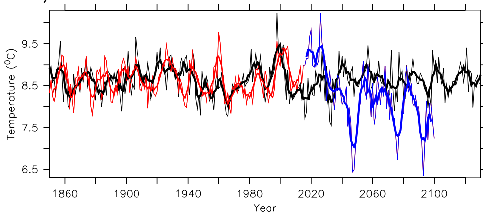
c) NorESM2-LM
