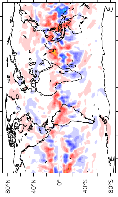
b) bcc-csm1-1
