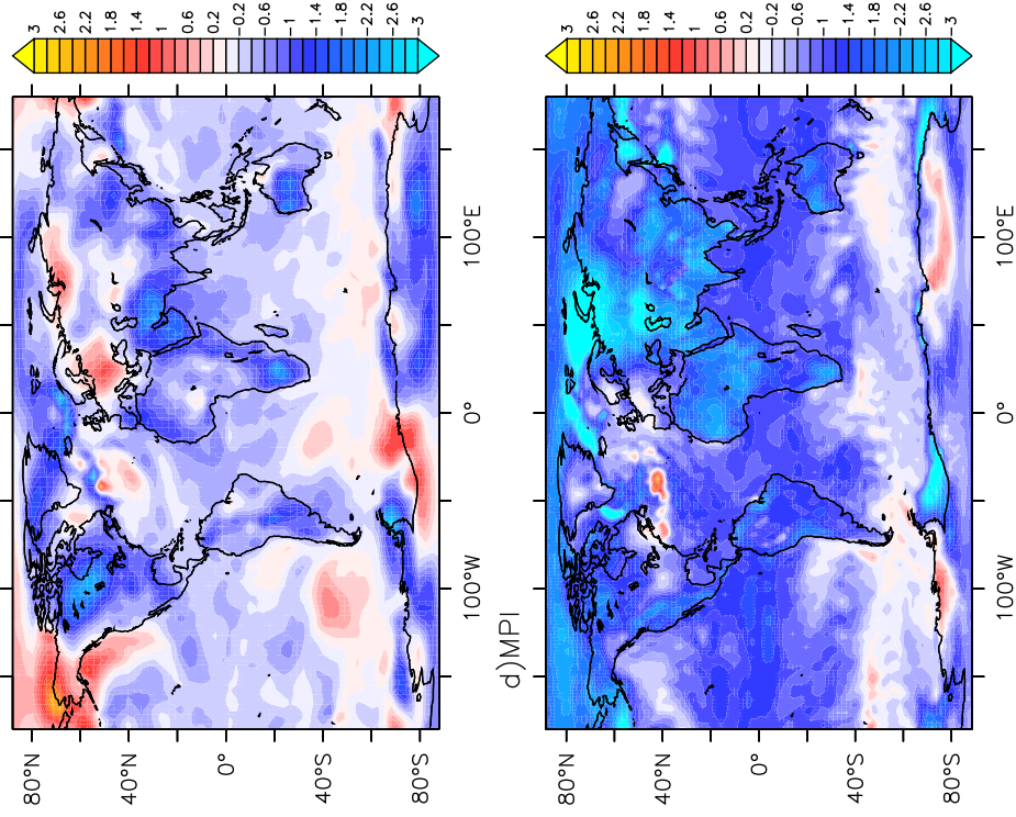
b) bcc-csm1-1
