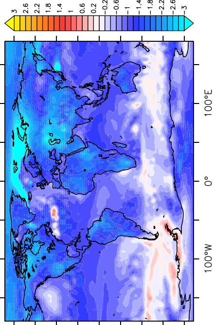
d) MPI
