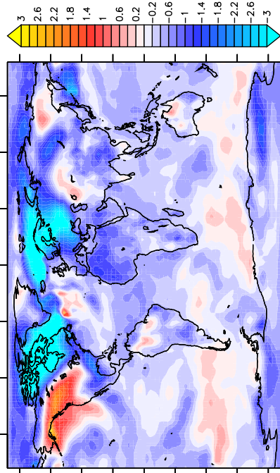
b) bcc-csm1-1
