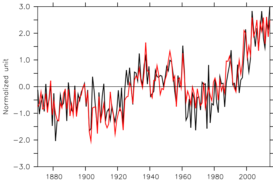
b) PC1 evolution ( r=0.89 )
