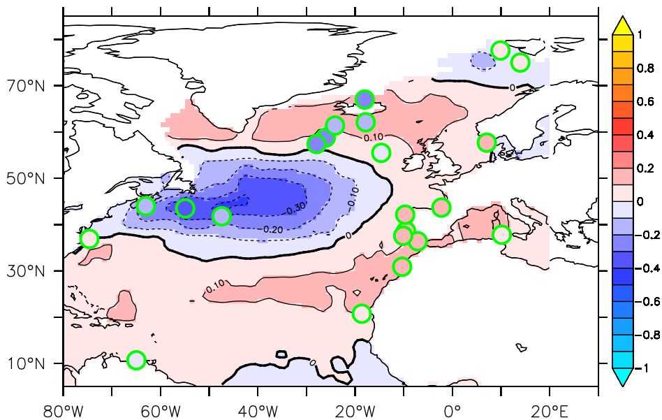
b) PC3 evolution ( r=0.4 )
