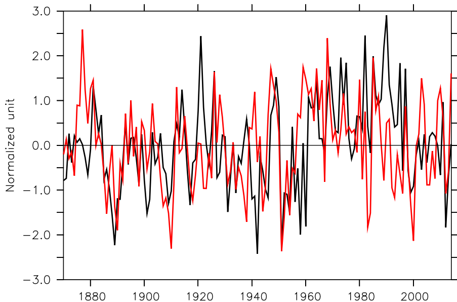
b) PC3 evolution ( r=0.4 )
