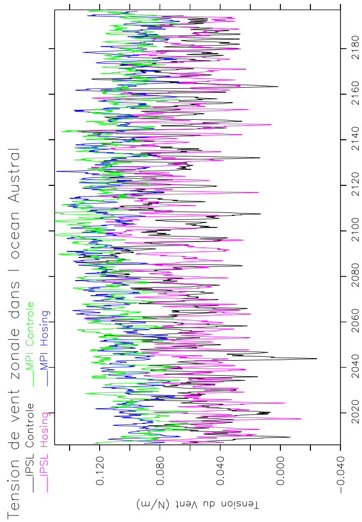
Localisation du vent dans l'hémisphère sud IPSL Control
