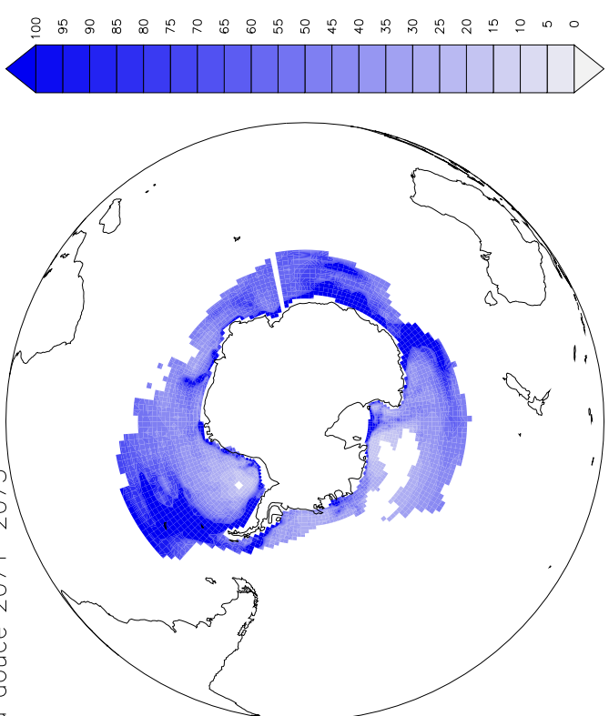
Flux d'eau douce 2071-2075
