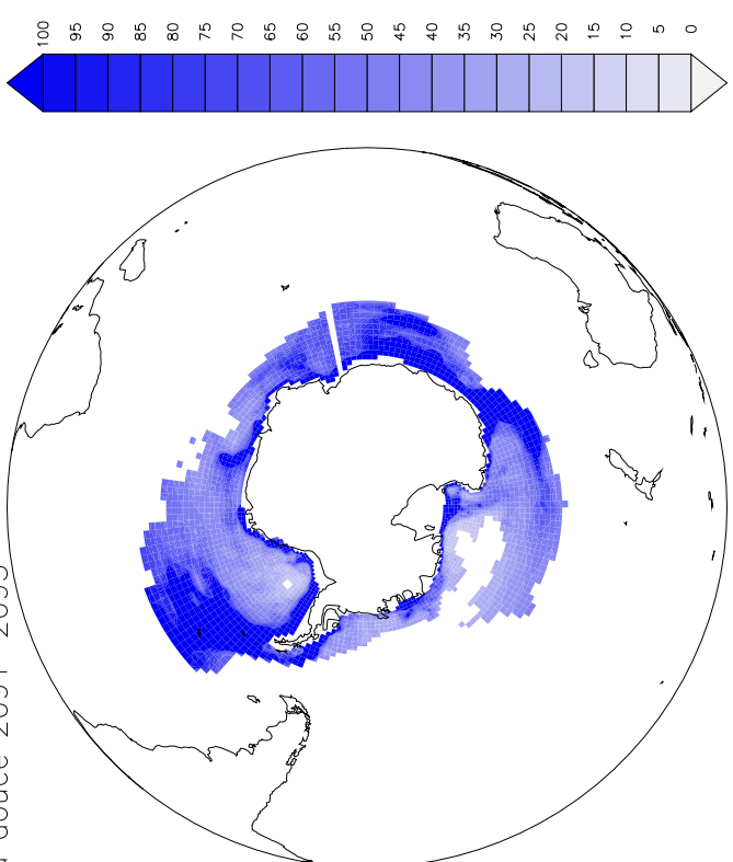
Flux d'eau douce 2091-2095
