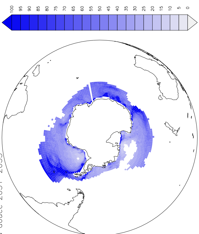
Flux d'eau douce 2031-2035
