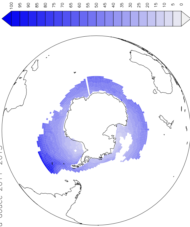
Flux d'eau douce 2011–2015
