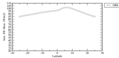
rsahzon
