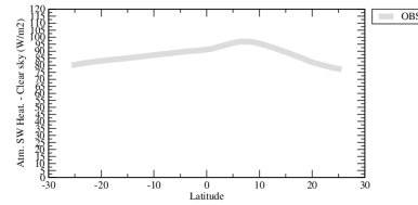
rsahcszon
