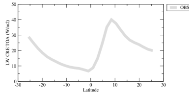
cretlzon
