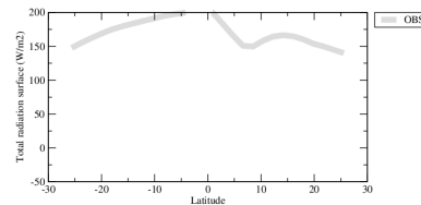
rtszon
