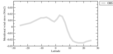
tauvzon
