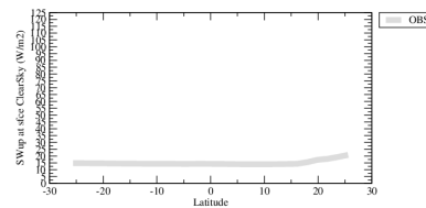
rsutcszon
