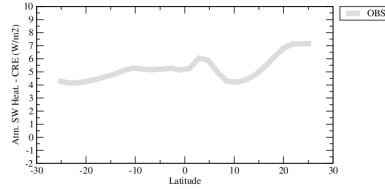
rsahcrezon
