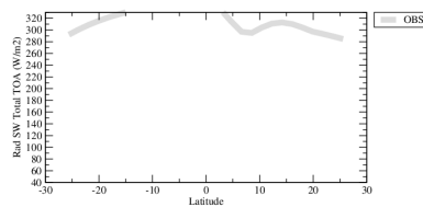
rsttzon
