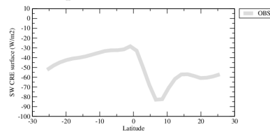
crestlzon
