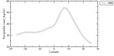
procezon
