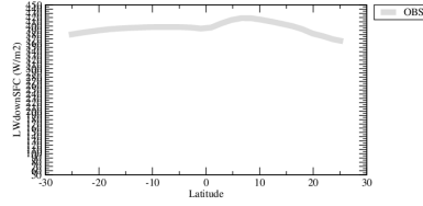
rldszon
