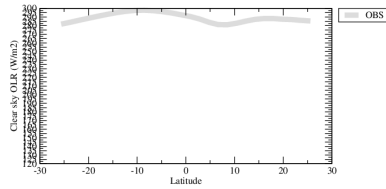
rlutcszon
