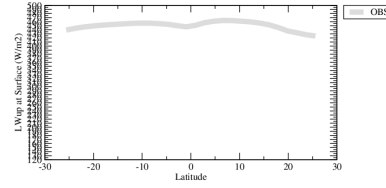
ruluszon
