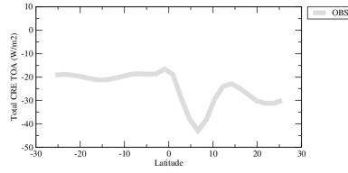
cretzon
