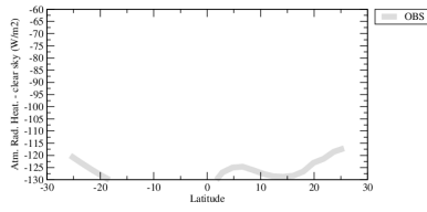
rahcszon
