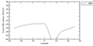
cretlzon
