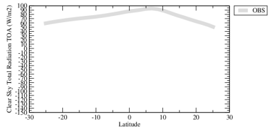
rttcszon
