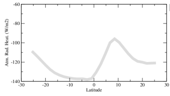
rahzon
