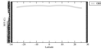
sstzon
