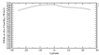
rsdscszon
