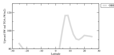
rsutzon
