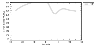
rsdszon
