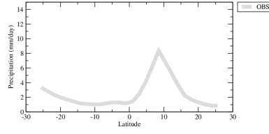
rahrefzon
