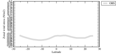
tauuzon
