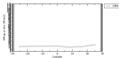
rsutzon
