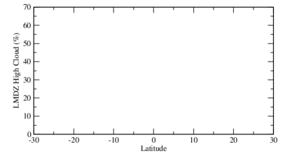
chlzon
