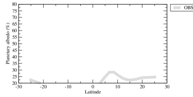
albtzon
