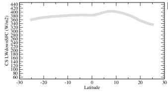
rldscszon
