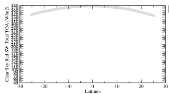
rsttcszon
