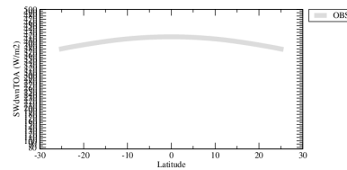
rsdtzon
