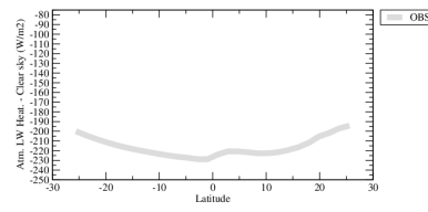
ralahcszon
