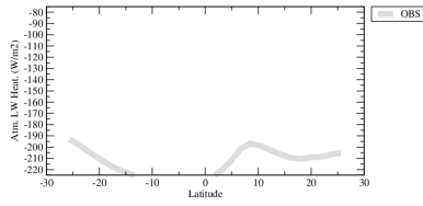
ralahzon
